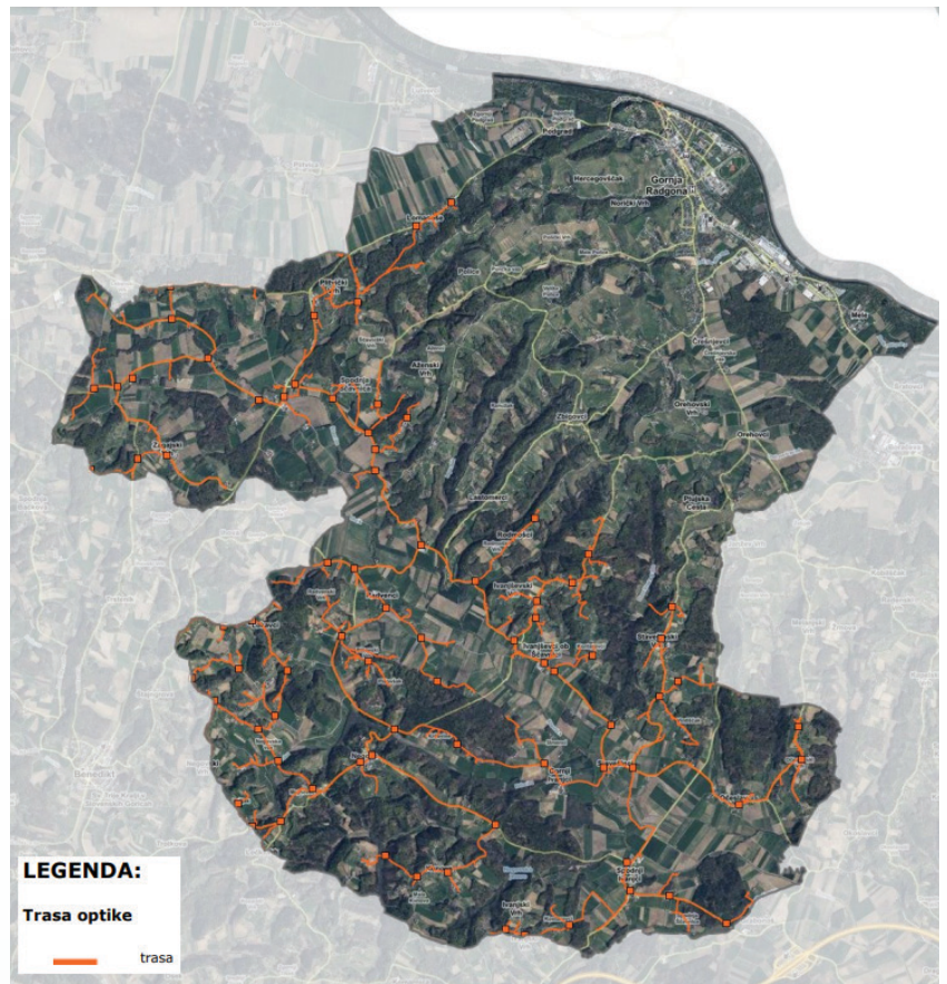
Simbolični prikaz trase OŠO, vir: PISO
