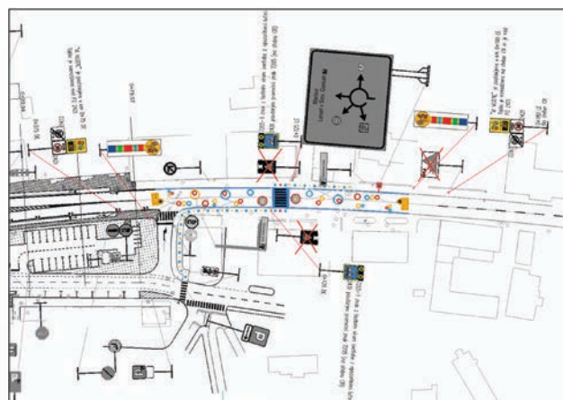
Načrt za izvedbo prehoda za pešce
